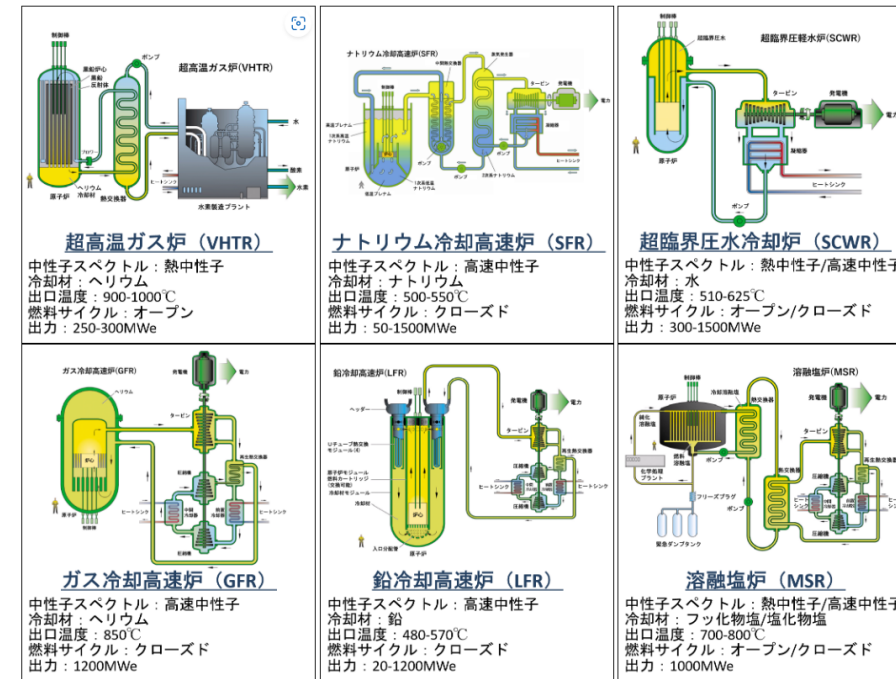
図2: GIFにおいて選定された第4世代原子力システム
